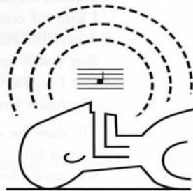
clarinet timbre
